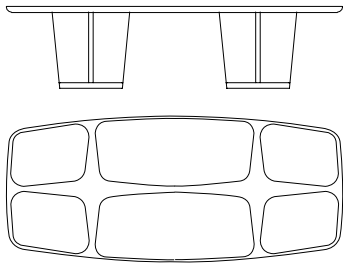
53134 Tavolo rettangolare in noce canaletto, inserti piano in sapelli Rectangular table in walnut canaletto, top with sapele inserts cm 300 x 130 x h 73 in 118 1/8 x 51 1/4 x h 28 3/4
