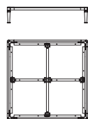
C 87011 Tavolino basso quadrato in acciaio, 4 doghe Low square coffee table in steel, 4 slats cm 110 x 110 x h 22 in 43 3/8 x 43 3/8 x h 8 5/8
