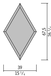
GA603G/MOD 4 Con bisellatura / with bevelled edge
